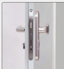
PZ-Schloss Klasse 3
