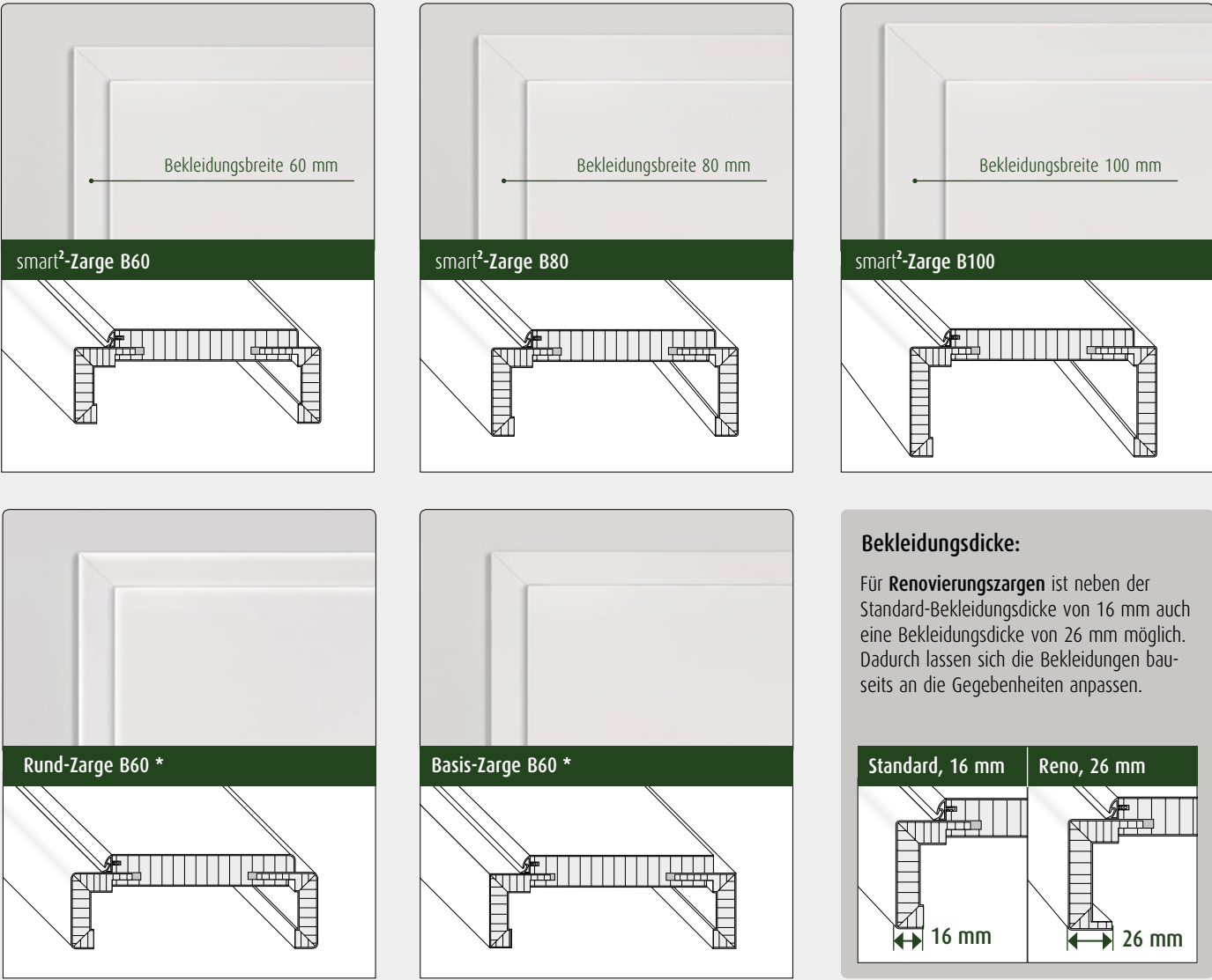
Zargentypen und Bekleidungsbreiten
