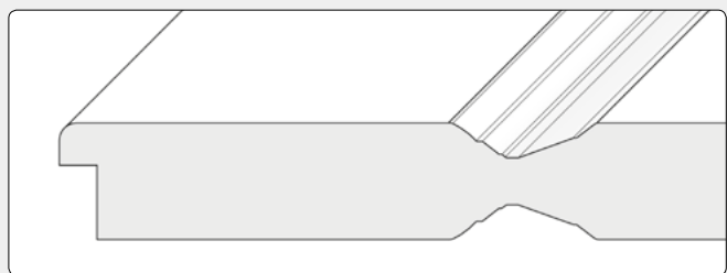
Türblatt mit liegenden Hohlprofilen, Einlage aus Röhrenspanplatten
