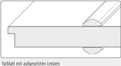
Türblatt mit aufgesetzten Leisten
