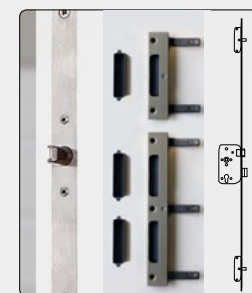
Dreifachverriegelung mit WE-Schließblech
