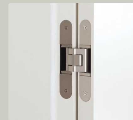
Das verdeckte »Tectus« Band sitzt im Tür- und Zargenfalz und ist bei geschlossener Tür nicht sichtbar.
