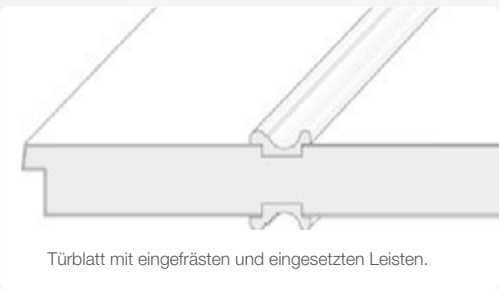
Querschnitt
