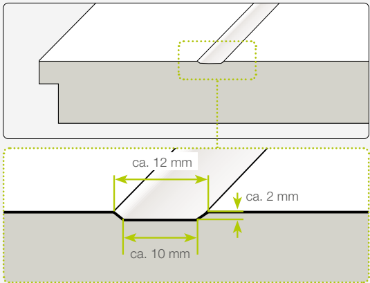
Lines Art | Querschnitt
