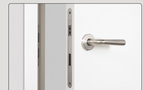
Das Schließblech ist bei geschlossener Tür nicht sichtbar, da das Schloss magnetisch verriegelt wird, ohne mechanischen Kontakt zum Schließblech.
